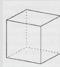
hexaëder zesvlak kubus
